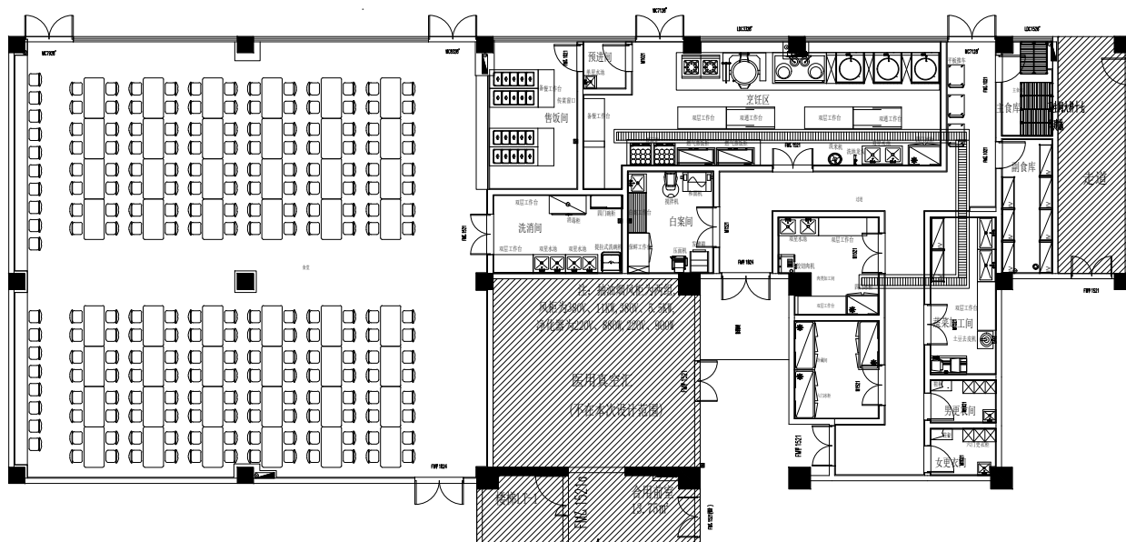
负一层平面图
