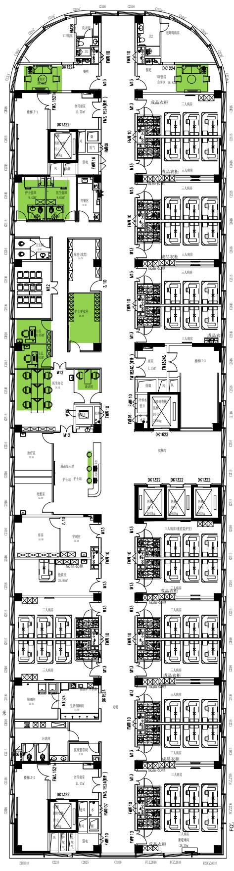
八层平面图
